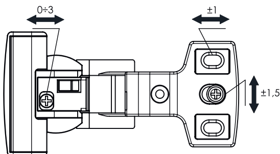
Schema Regolazioni Adjustments Diagram
